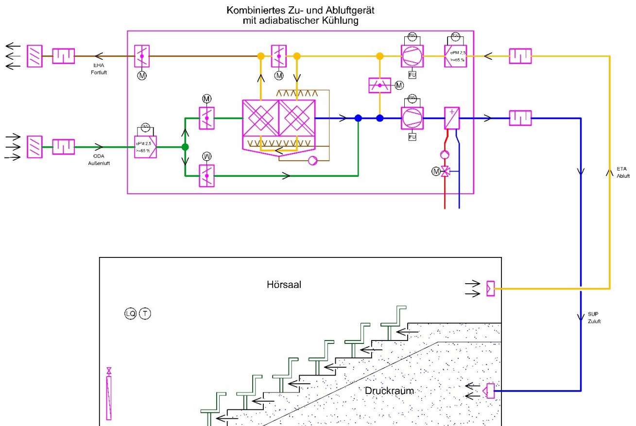
Abbildung 2: Beispiel 1 einer RLT-Anlage für Hörsäle
