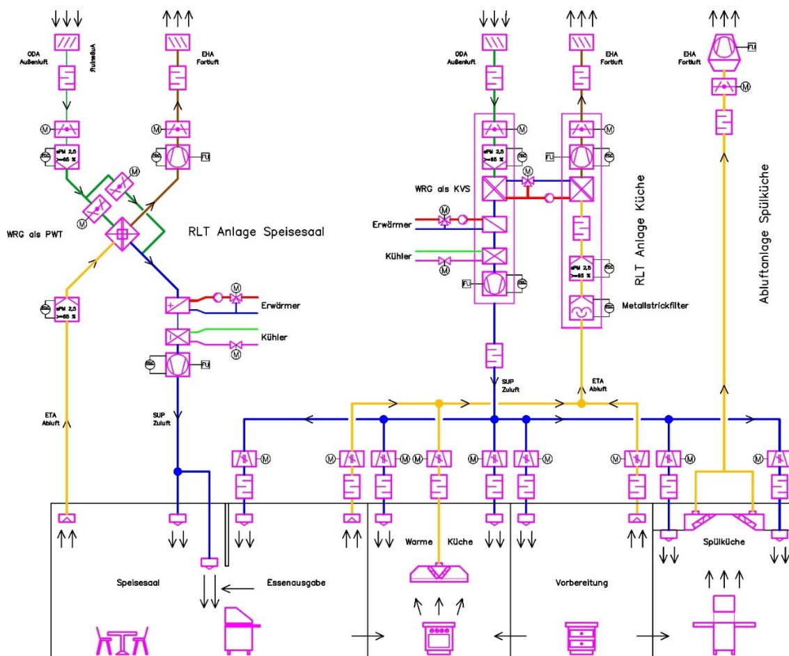
Abbildung 6: Beispiel einer RLT-Anlage für eine Küche
