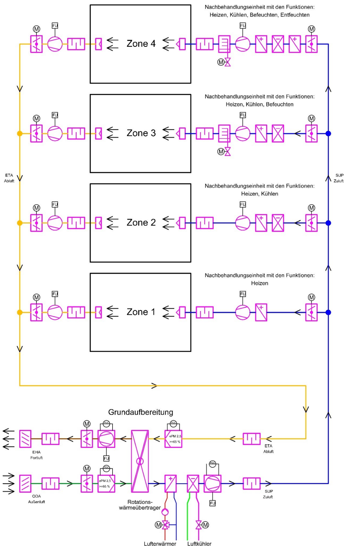
Abbildung 5: Beispiel einer RLT-Anlage als großes Versorgungssystem mit Mehrzonenanlage
