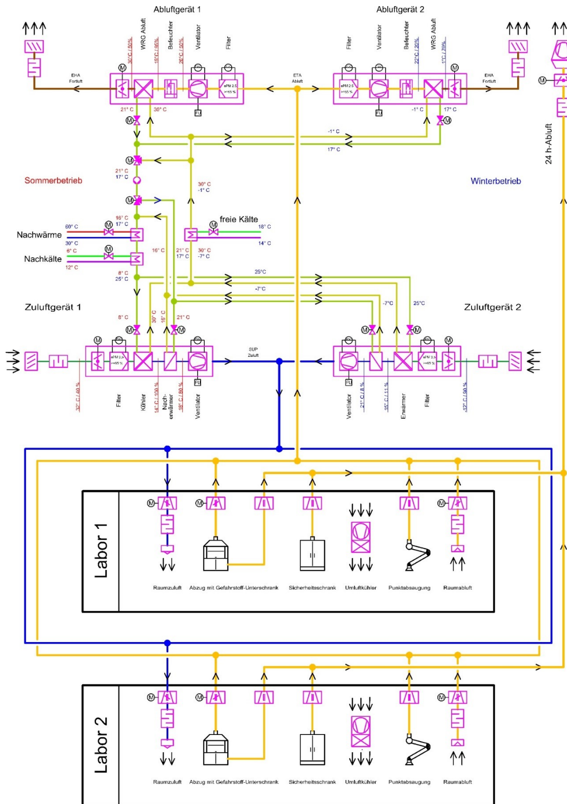
Abbildung 4: Beispiel einer RLT-Anlage für Laborgebäude
