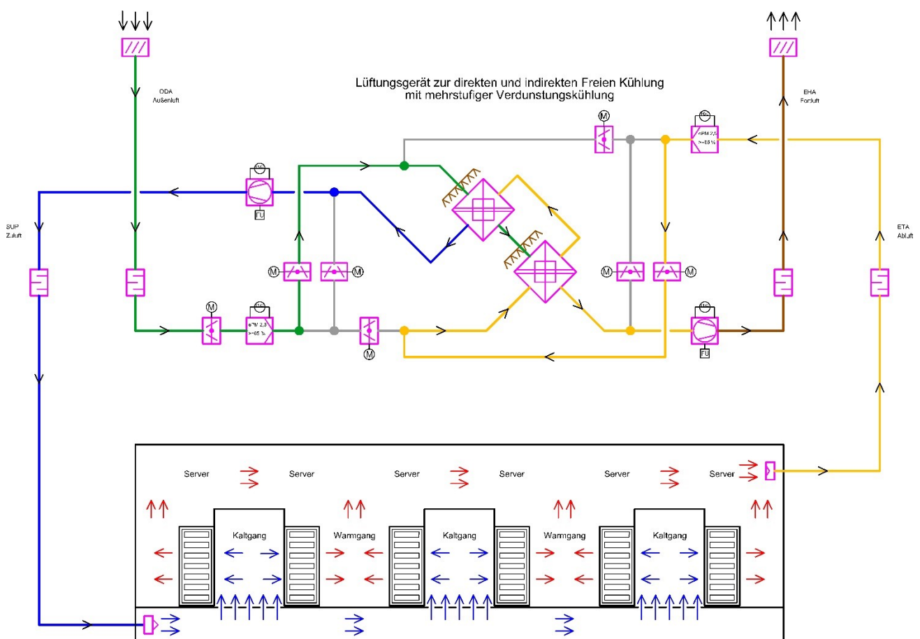
Abbildung 7: Beispiel einer RLT-Anlage für ein Rechenzentrum
