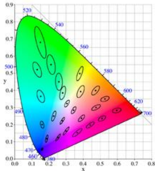
Abbildung 12: MacAdam-Ellipsen, zur Verdeutlichung 10-fach vergrößert.
